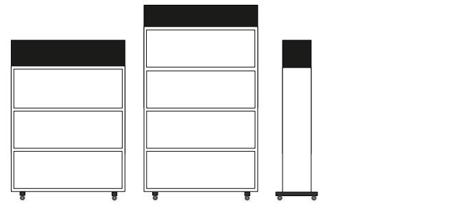
B: 1200 mm H: 1370 mm med hylla inkl. hjul art.nr 15-1213-H B: 1200 mm H: 1720mm med hylla inkl. hjul art.nr 15-1217-H Stomme djup: 345 mm Fot: 550×55×45 mm H100 mm inkl. hjul
