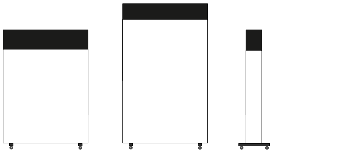
B: 1200 mm H: 1200 mm inkl. hjul art.nr 15-1212 B: 1200 mm H: 1600 mm inkl. hjul art.nr 15-1216 Stomme djup: 225 mm Fot: 550×55×45 mm H: 105 mm inkl. hjul
