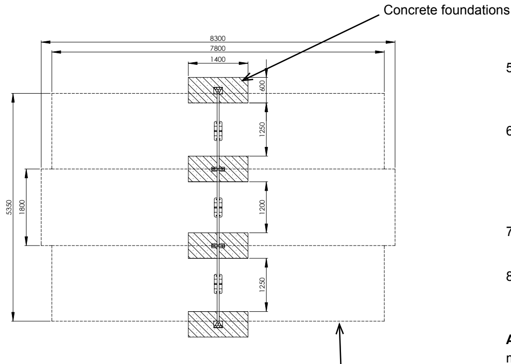
Diagram 3: Top view „patis3“
