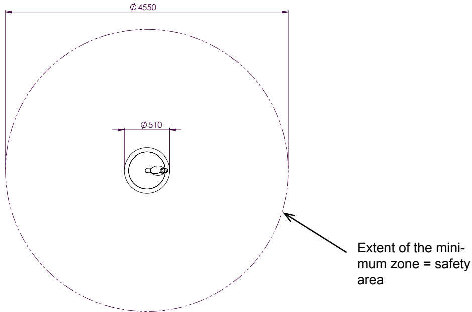
Diagram 3: Top view „cita“
