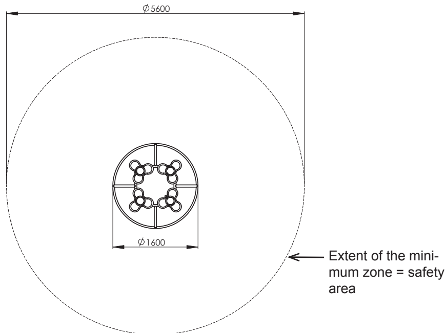
Diagram 3: Top view „circulus4“
