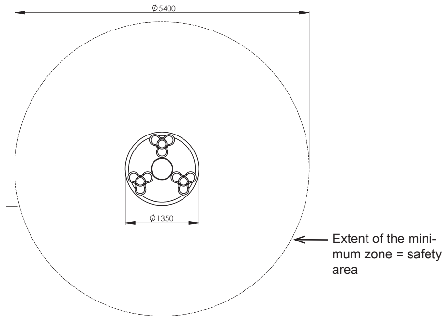
Diagram 3: Top view „circulus3“
