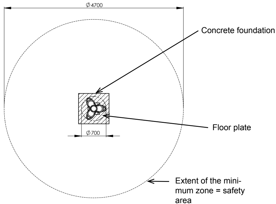
Diagram 3: Top view „circulus1“
