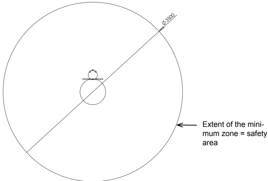
Diagram 3: Top view „Lilly“
