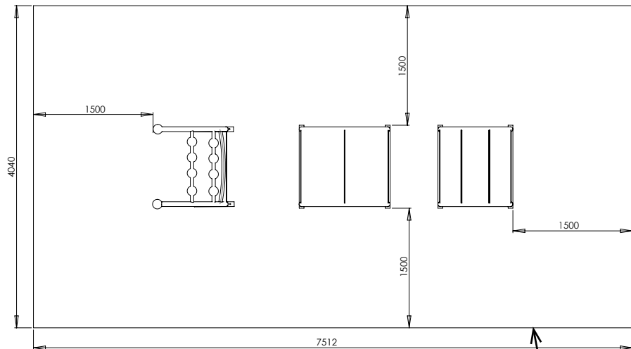
Diagram 3: Top view „Erika“
