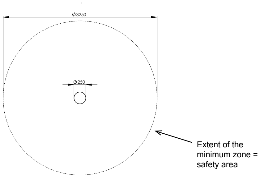
Diagram 3: Top view „pinna2“
