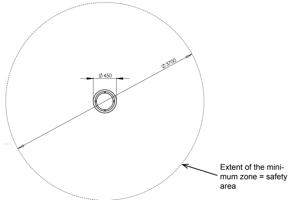
Diagram 3: Top view „pinna“
