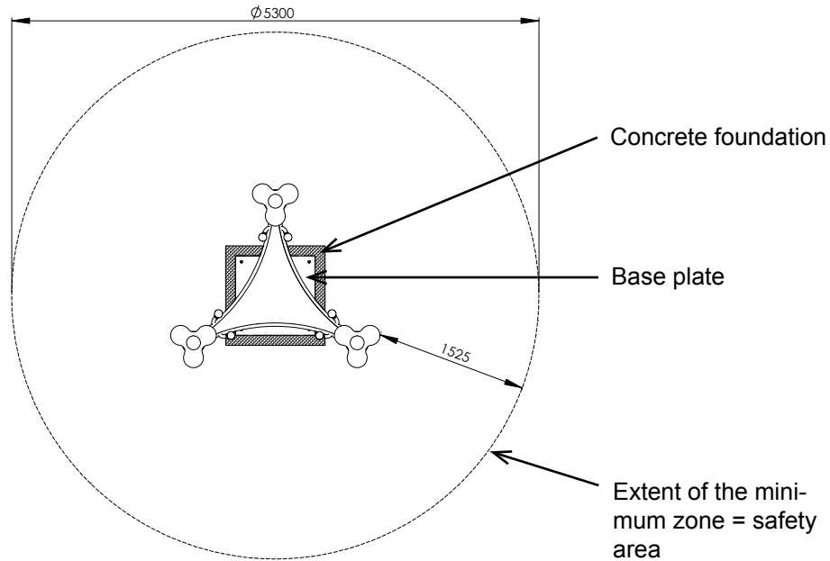
Diagram 3: Top view „papilio3“
