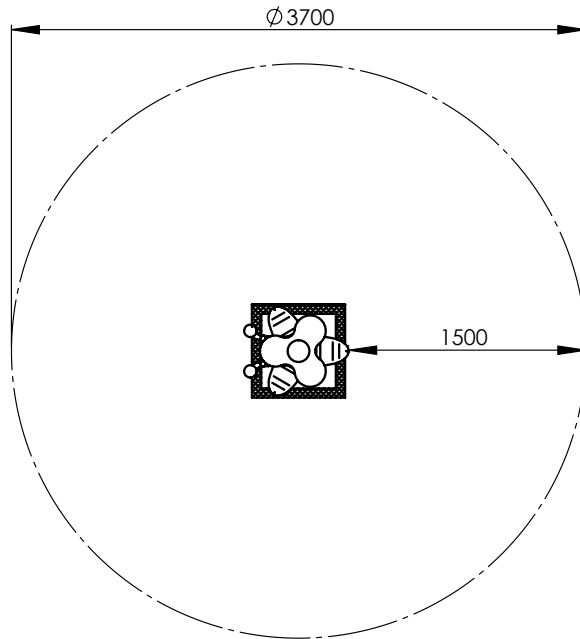
Diagram 3: Top view „papilio1“
