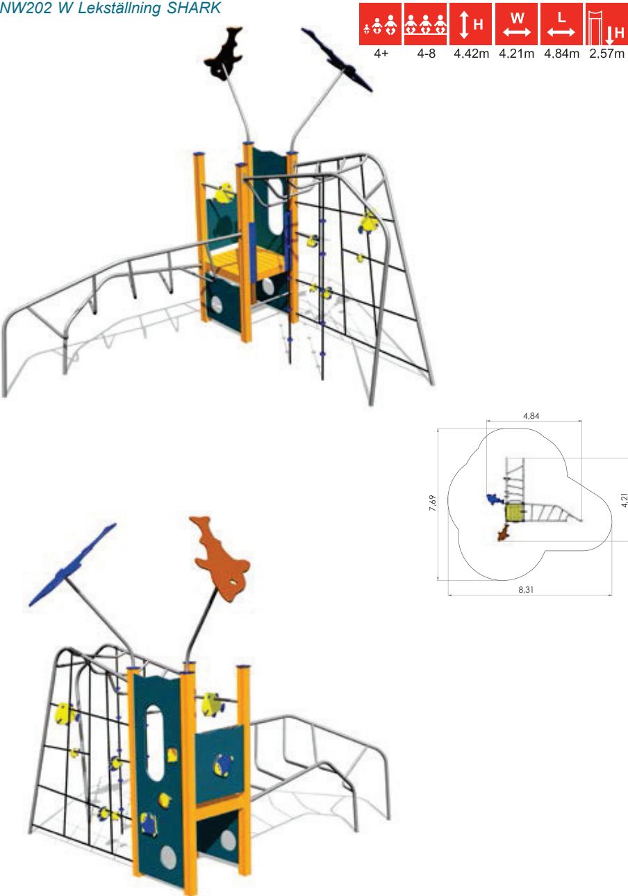
NW202 W Lekställning SHARK
