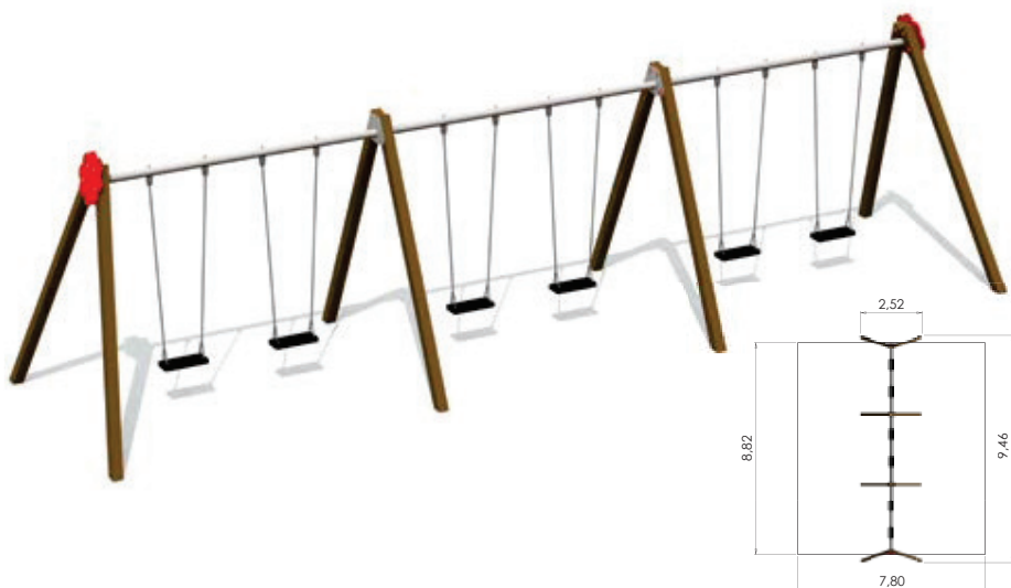
K009 Gungställning BELL-FLOWER 6 platser
