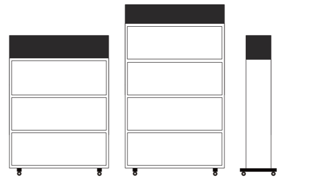
Stomme djup: 225 mm Fot: 550x55x45 mm H: 105 mm inkl. hjul
