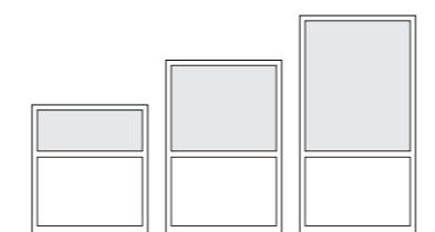
Offizz 800 x 1100 Offizz 800 x 1500 Offizz 800 x 1900 djup 70
