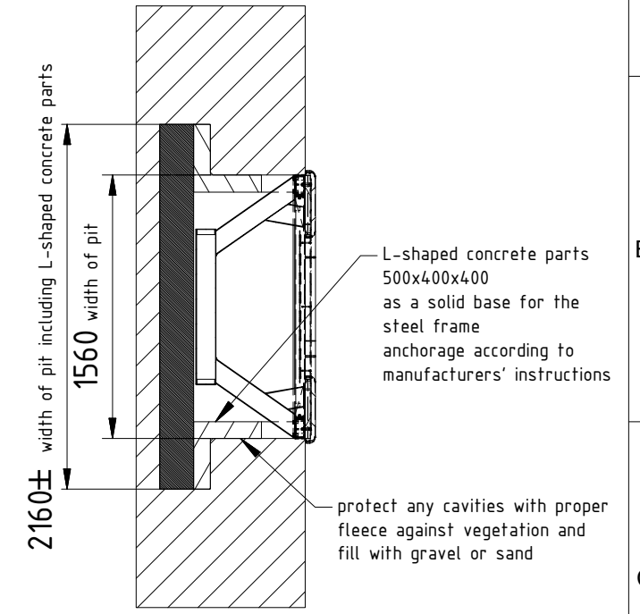
A-A ( 1 : 40 )
