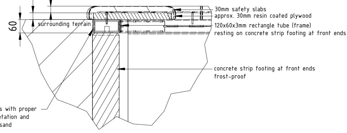
C ( 1 : 10 )
