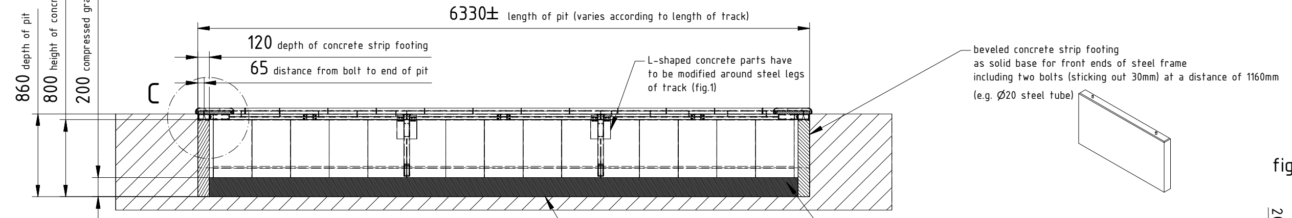
C ( 1 : 10 )
