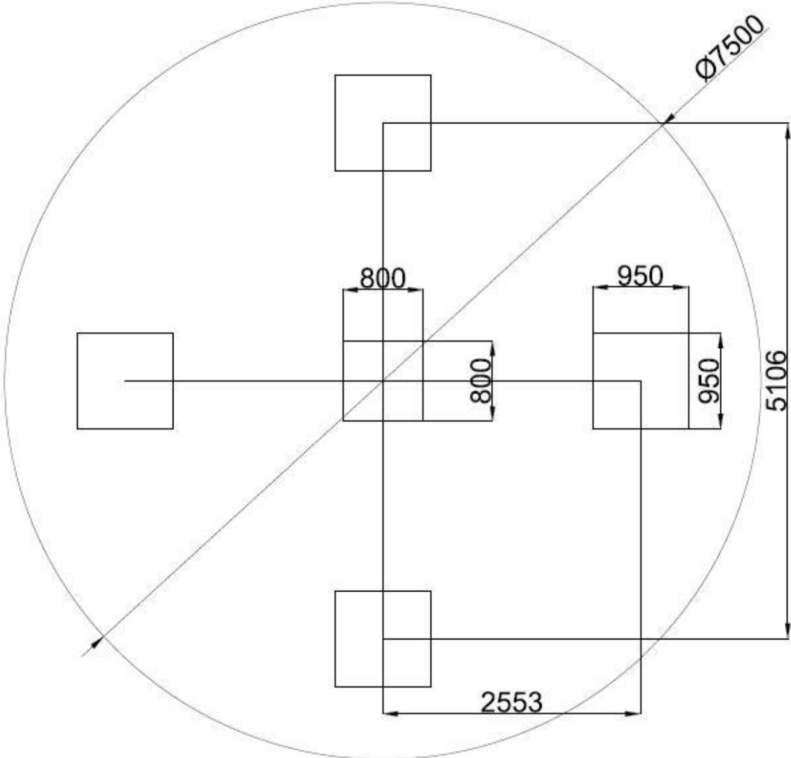
Ritning 1: Fundamentplan
